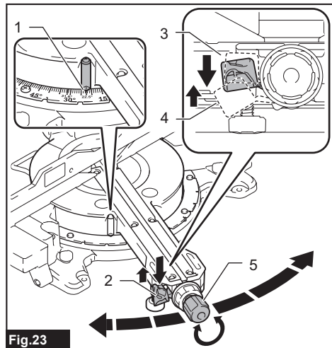
► 1. Ángulo del tope de seguridad 2. Palanca de liberación 3. Posición bloqueada 4. Posición desbloqueada 5. Perilla
