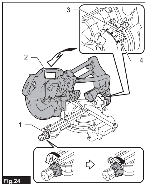
► 1. Selector de perilla 2. Empuñadura 3. Marcador 4. Escala del ángulo de bisel
