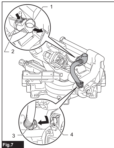
► 1. Codo 2. Botón de bloqueo 3. Manguito 4. Puerto
